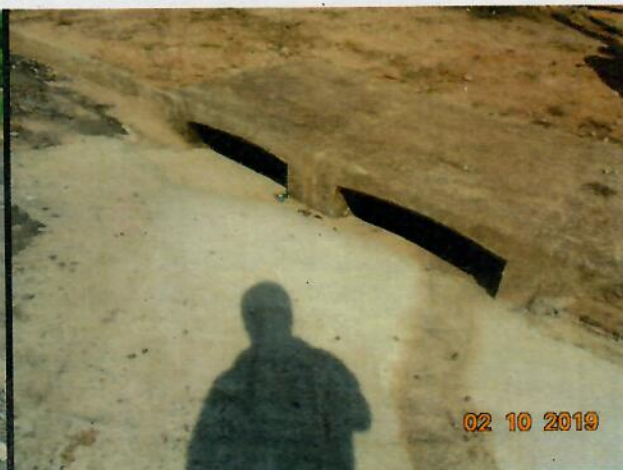
Foto 12 – Boca de lobo dupla existente na Rua Cedro, que recebe contribuição do Sarjetão da Foto 13.
